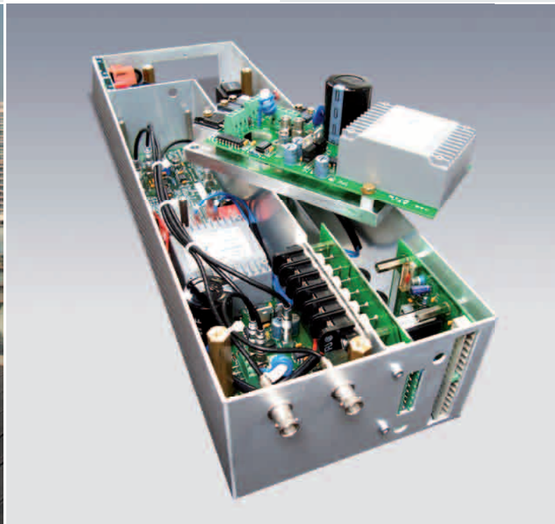
Automatisierungstechnik – Zentralsterelektronik für Laserbearbeitung
